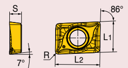
Правосторонняя (XCGT 0401)
