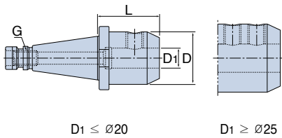
DIN 2080 DIN 6359 / DIN 1835 Форма В
