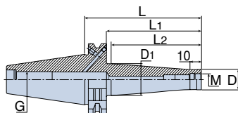
DIN 69871 Форма ADB
