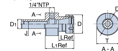
Цилиндрический хвостовик DIN 6499
