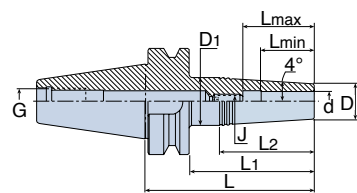
BT MAS 403 Форма AD
