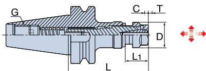
BT MAS - 403 Форма А DIN 6499 GTI
