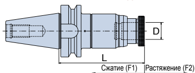
BT MAS-403 Форма А ПАТРОН ДЛЯ МЕТЧИКОВ
