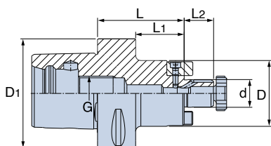
C-АДАПТЕРЫ (ISO 26623-1) ISO 3937
