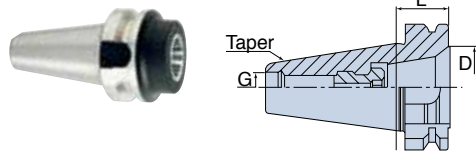
BT MAS-403 Форма AD T-CLICK
