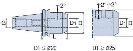
DIN 69871 Форма AD DIN 6359/DIN1835 Форма E
