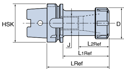
HSK DIN 69893 Форма A
