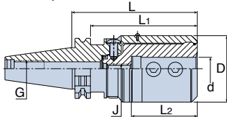
DIN69871 Форма AD
