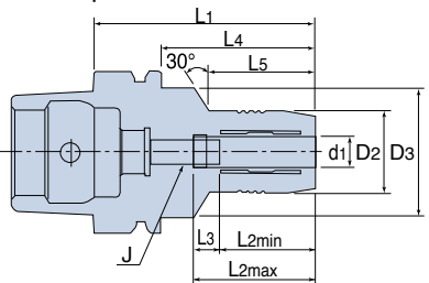
DIN 69893 Форма Е
