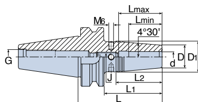
BT MAS-403 Форма AD
