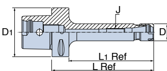
С-АДАПТЕРЫ (ISO 26623-1) ER DIN6499
