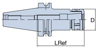
BT MAS-403 Форма AD TSK
