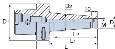
C-АДАПТЕРЫ (ISO 26623-1) T-FLEXTEC
