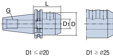
DIN 69871 Форма AD DIN 6359/DIN1835 Форма B
