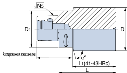
C-АДАПТЕРЫ (ISO 26623-1) Заготовка
