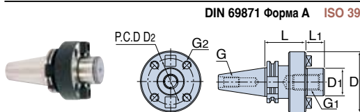
DIN 69871 Форма А ISO 3937
