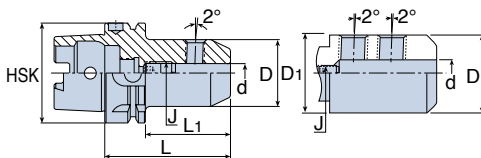
DIN 69893 Форма A DIN 6355/DIN 1835 Форма E
