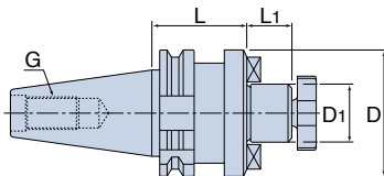
DIN 69871 Форма А
