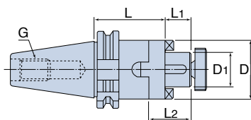
DIN 69871 Форма А
