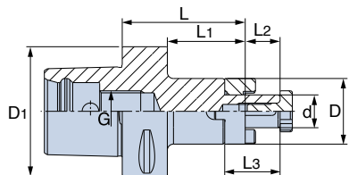
C-АДАПТЕРЫ (ISO 26623-1) DIN6358
